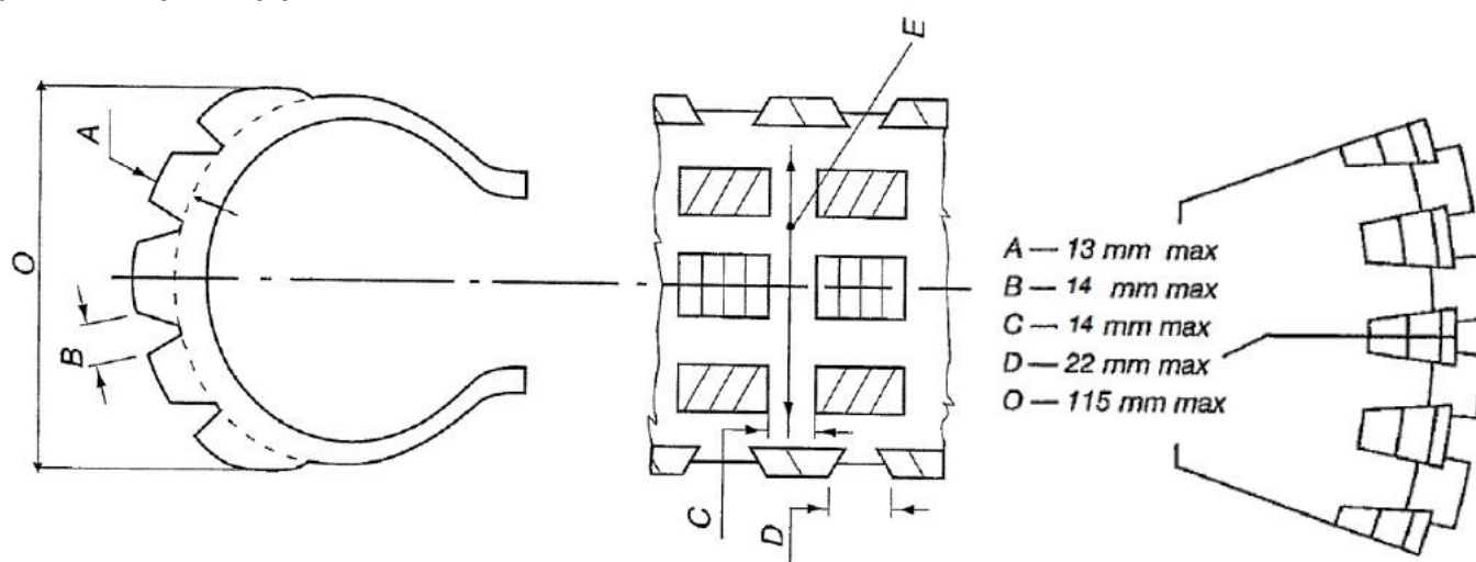
Obrázok 3: Rozmery pneumatiky
